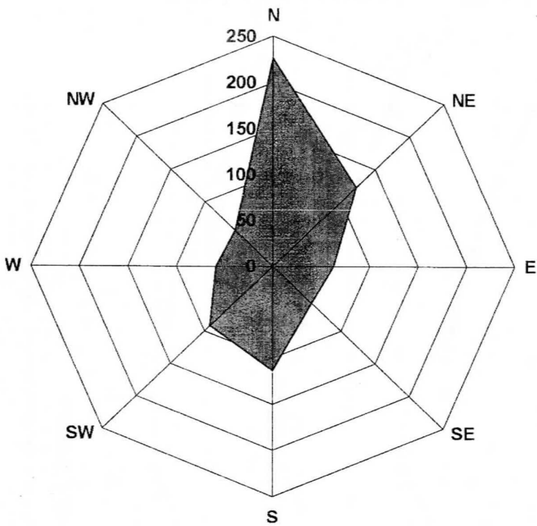
Figura 6: Frecuencia media anual de direcciones del viento entre 1941 y 1990
